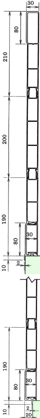
【組立図】
