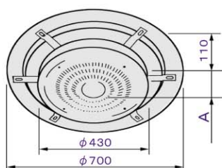
寸図仕様
